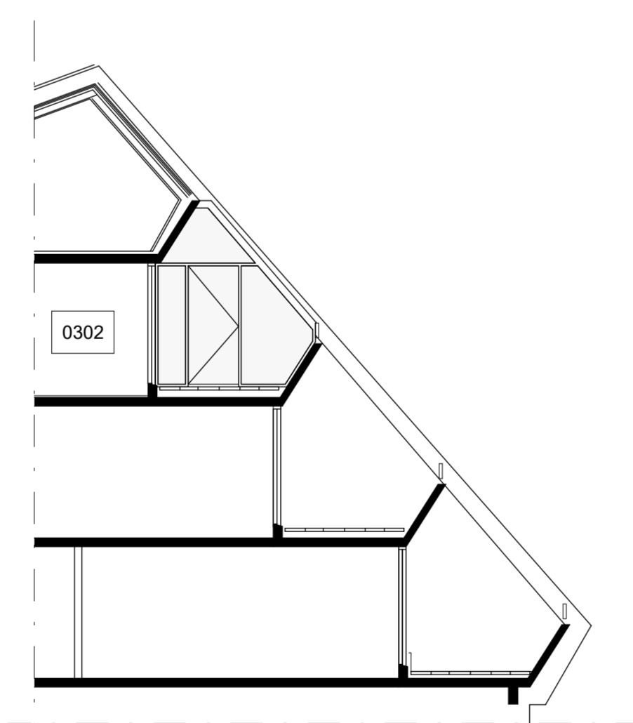
2 Snið 1:100
