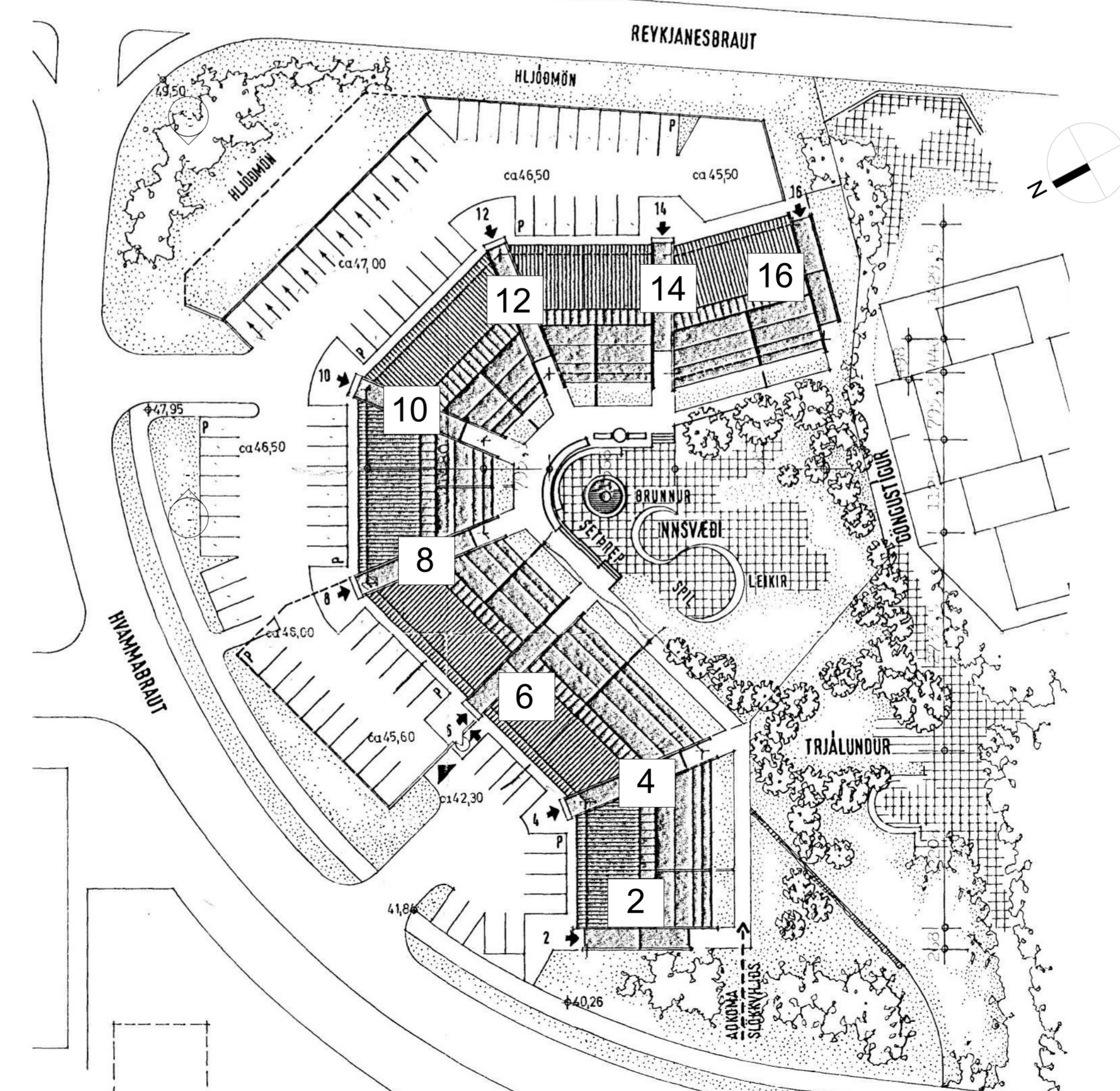
3 Afstöðumynd 1:500
